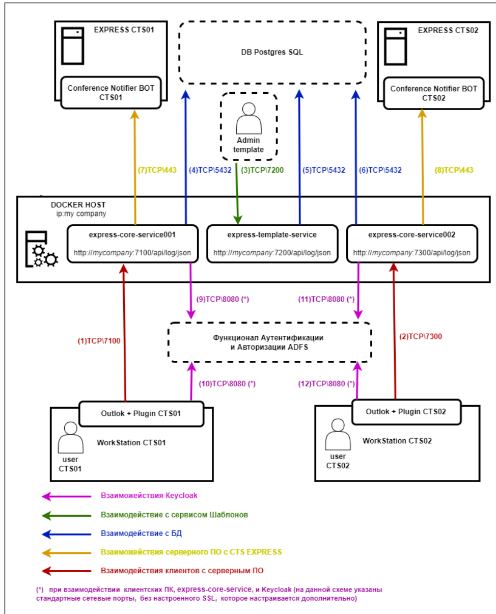
Рисунок 3. Типовая схема: 2 CTS, 2 express-core-service, 1 express-template-service
