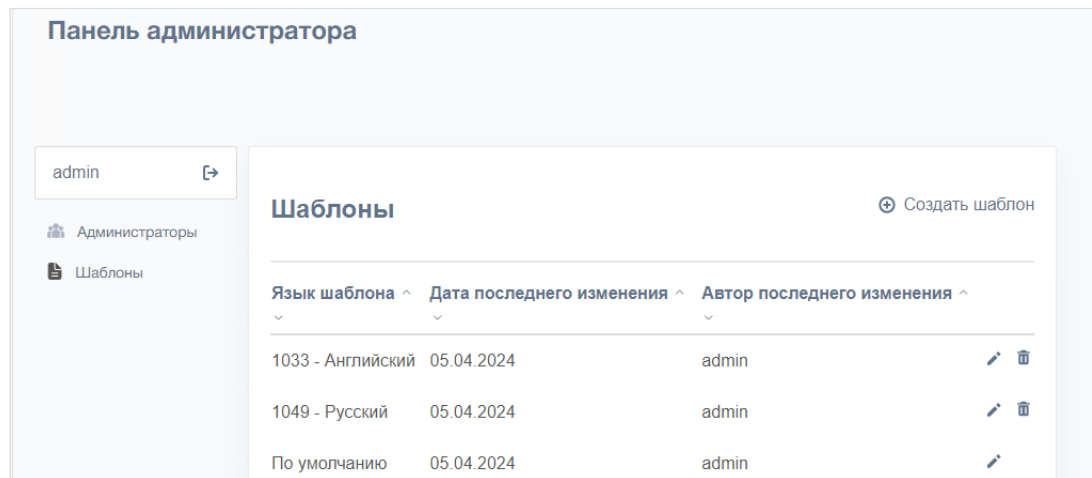
Рисунок 16. Раздел «Шаблоны»
