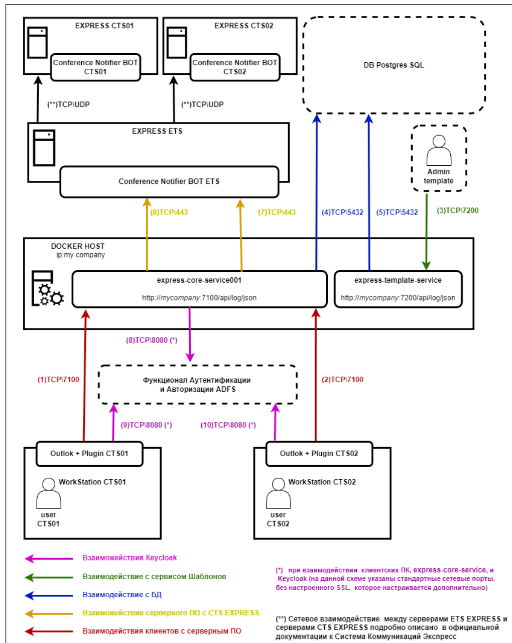
Рисунок 4. Типовая схема: 1 ETS, 2 CTS, 1 express-core-service, 1 express-template-service
