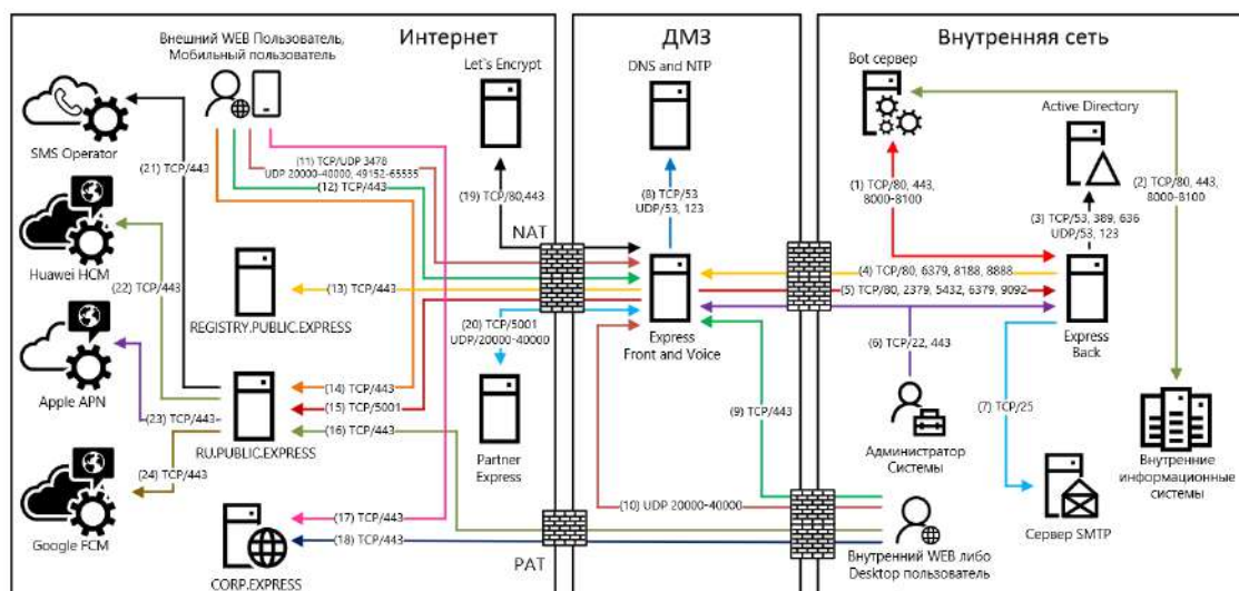
Рисунок 2. Типовая схема развертывания разделенного CTS (Front/Back)
